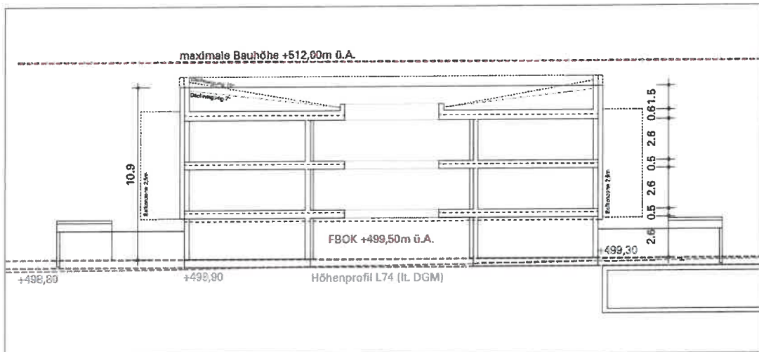
Systemschnitt nördliches Baufeld o. M. (Stand: 22.07.2024)
