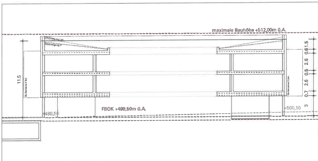
Systemschnitt südliches Baufeld o. M. (Stand: 22.07.2024)
