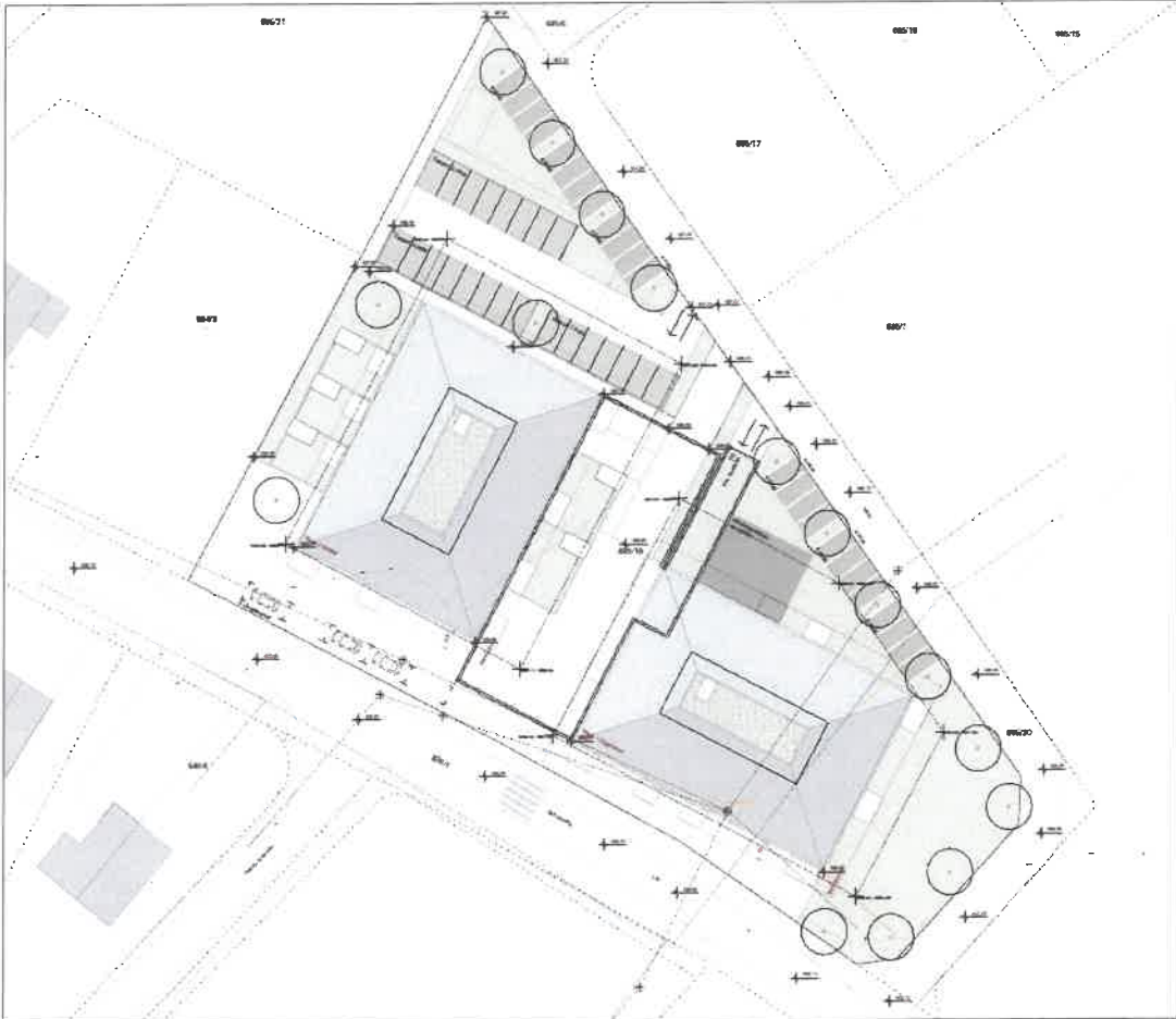
Lageplan o. M. (Stand: 27.08.2024)
